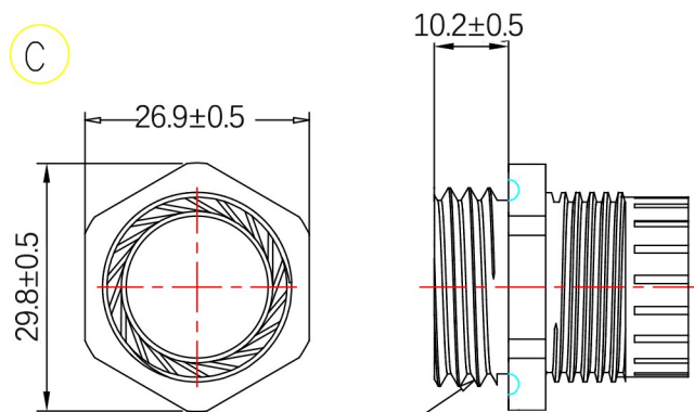
本体 Body
