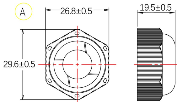
迫紧头 SealingNut
