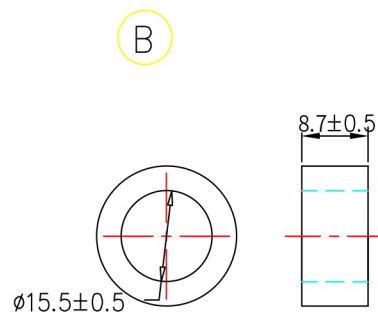
夹紧圈 Seal
