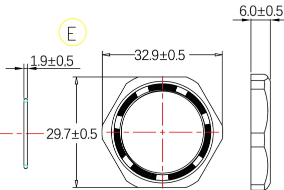
螺母 Lock Nut
