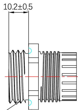
夹紧爪 Claw
