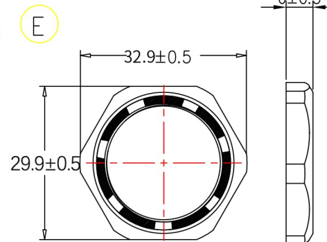
螺母 Lock Nut
