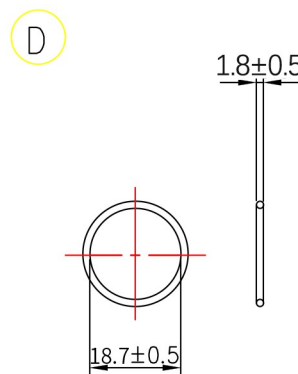
防水圈 Washer
