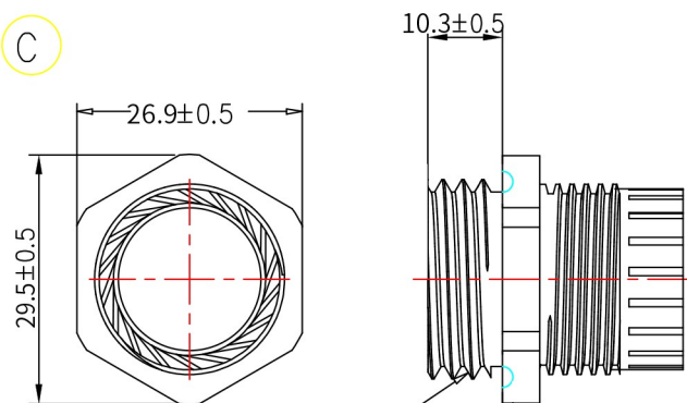
本体 Body
