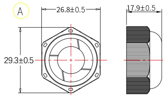
迫紧头 SealingNut
