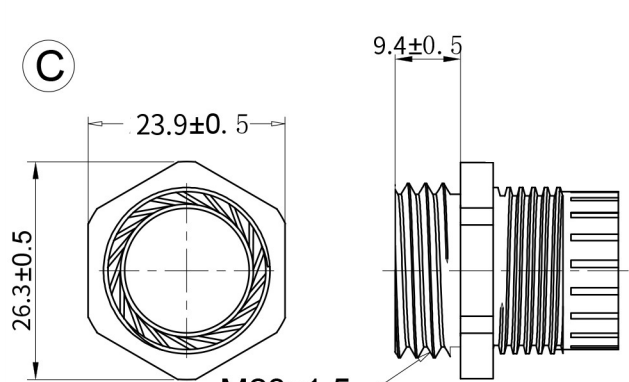
本体 Body
