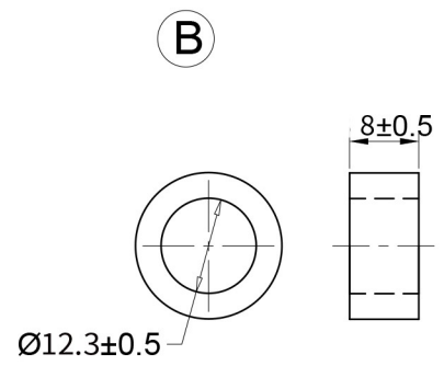
夹紧圈 Seal
