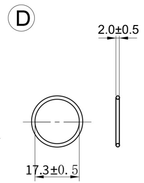
防水圈 Washer
