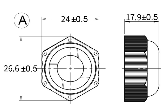
迫紧头 SealingNut
