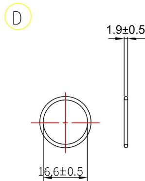
防水圈 Washer
