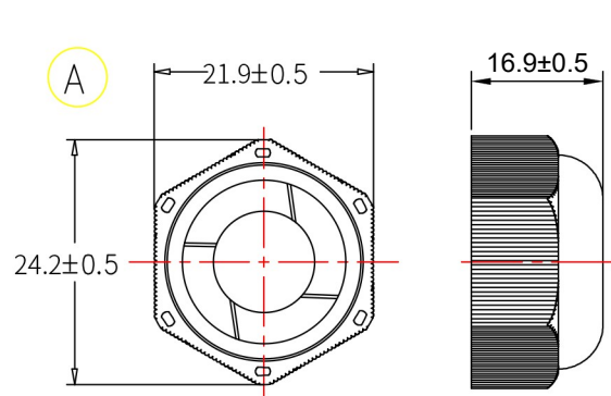
迫紧头 SealingNut
