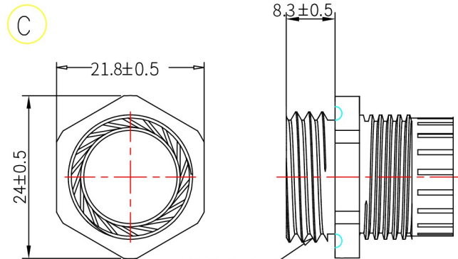
本体 Body
