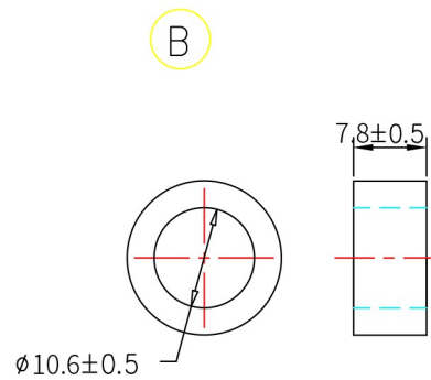
夹紧圈 Seal
