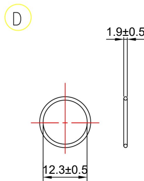
防水圈 Washer
