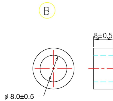
夹紧圈 Seal
