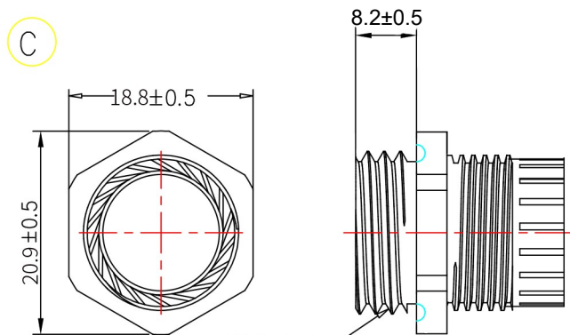
本体 Body
