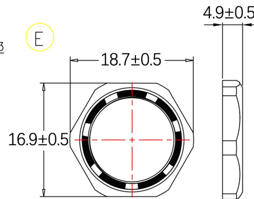
螺母 Lock Nut
