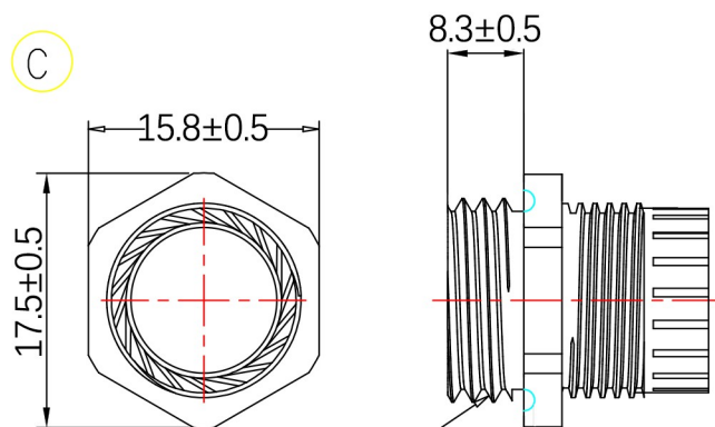
本体 Body
