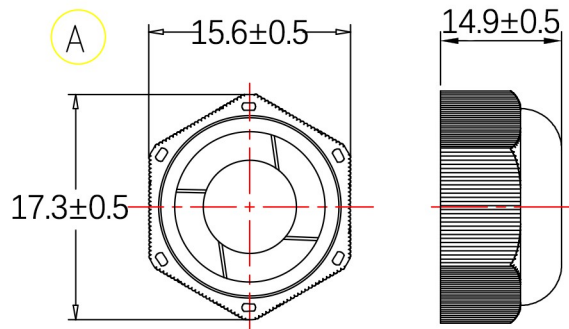
迫紧头 SealingNut
