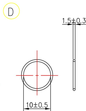
防水圈 Washer
